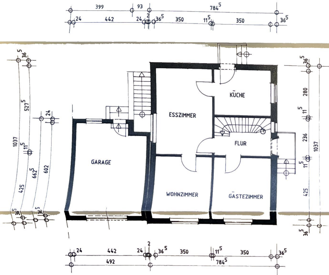
ERDGESCHOSS M. 1 : 100
