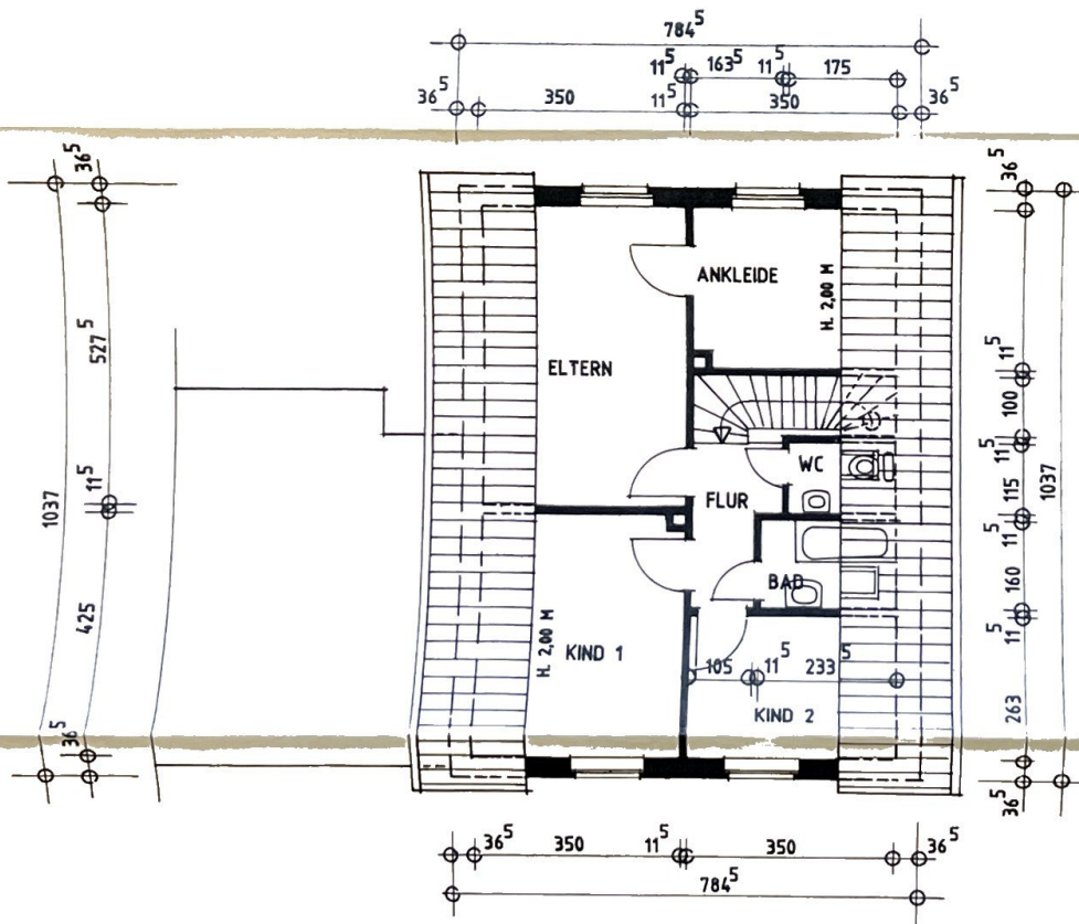
DACHGESCHOSS M. 1 : 100
